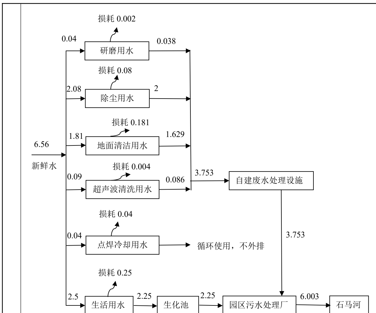
图 2.7-1 本项目水平衡图 单位: m 3 /d
