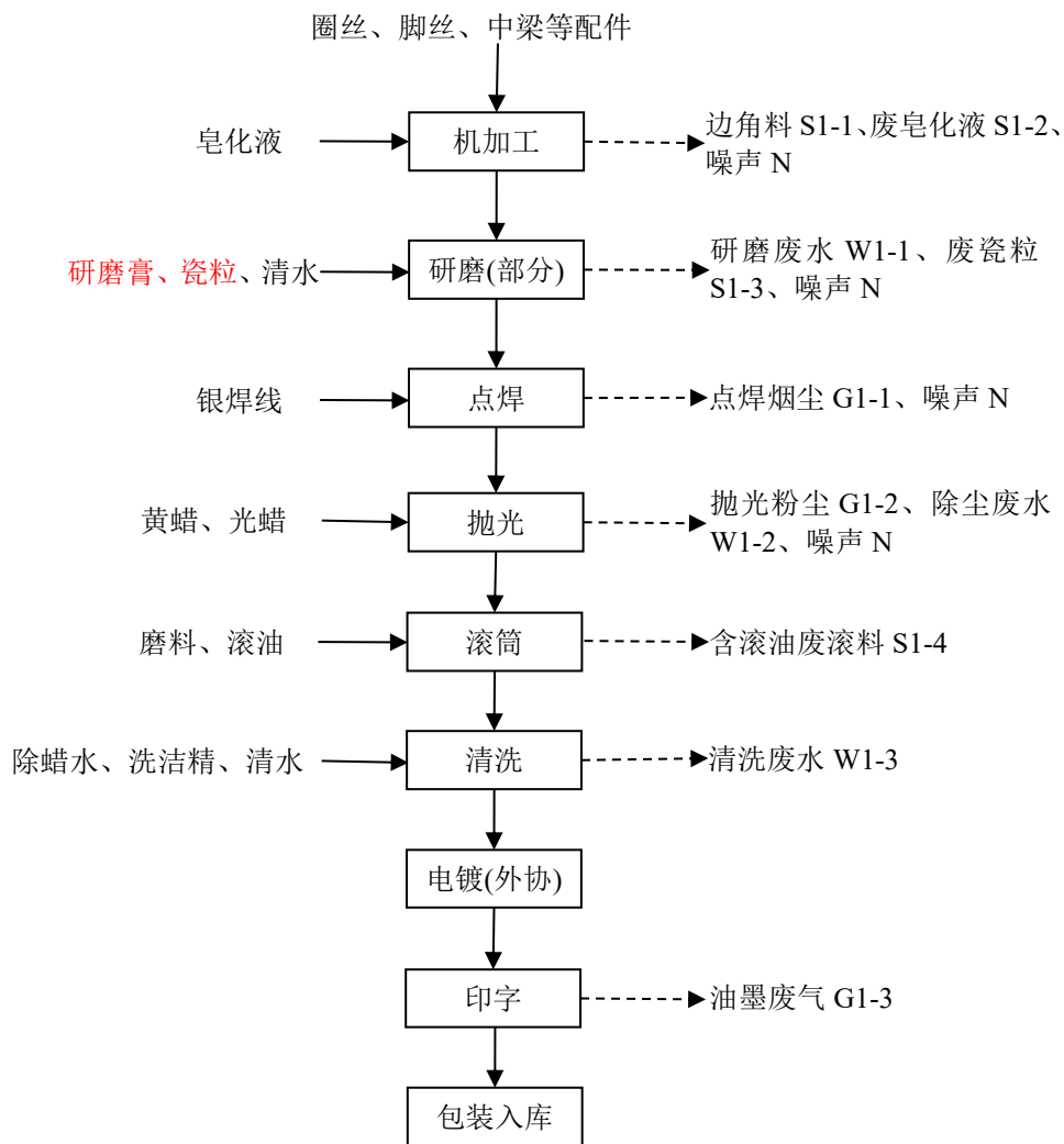
图 2.12-1 金属镜架及钛架生产工艺流程及产污环节图
